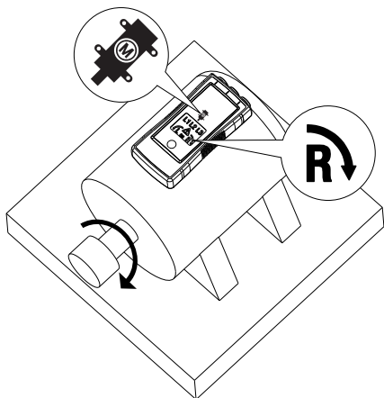
Figure 2 : Rotation moteur
